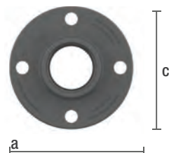
REF: Brida Van Stone de 2"
