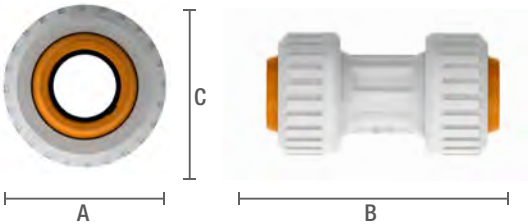
REF: Unión de reparación 1/2"
