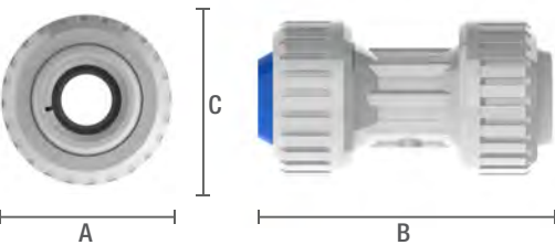
REF: Unión de Transición PE 20mm a Cobre 16mm
